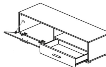
Тумба RTV1K1S L 140/35/45 шир./выс./глуб.
